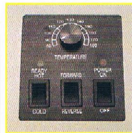
มีปุ่มปรับอุณหภูมิ มีปุ่มปรับเลือกเคลือบร้อน-เย็น มีปุ่มปรับเดินหน้า-ถอยหลัง
