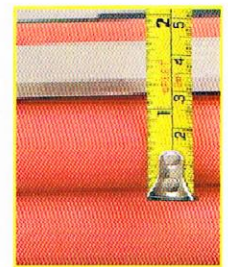
ลูกกลิ้งความร้อน จำนวน 4 ลูก เส้นผ่าศูนย์กลาง 20 มม.
